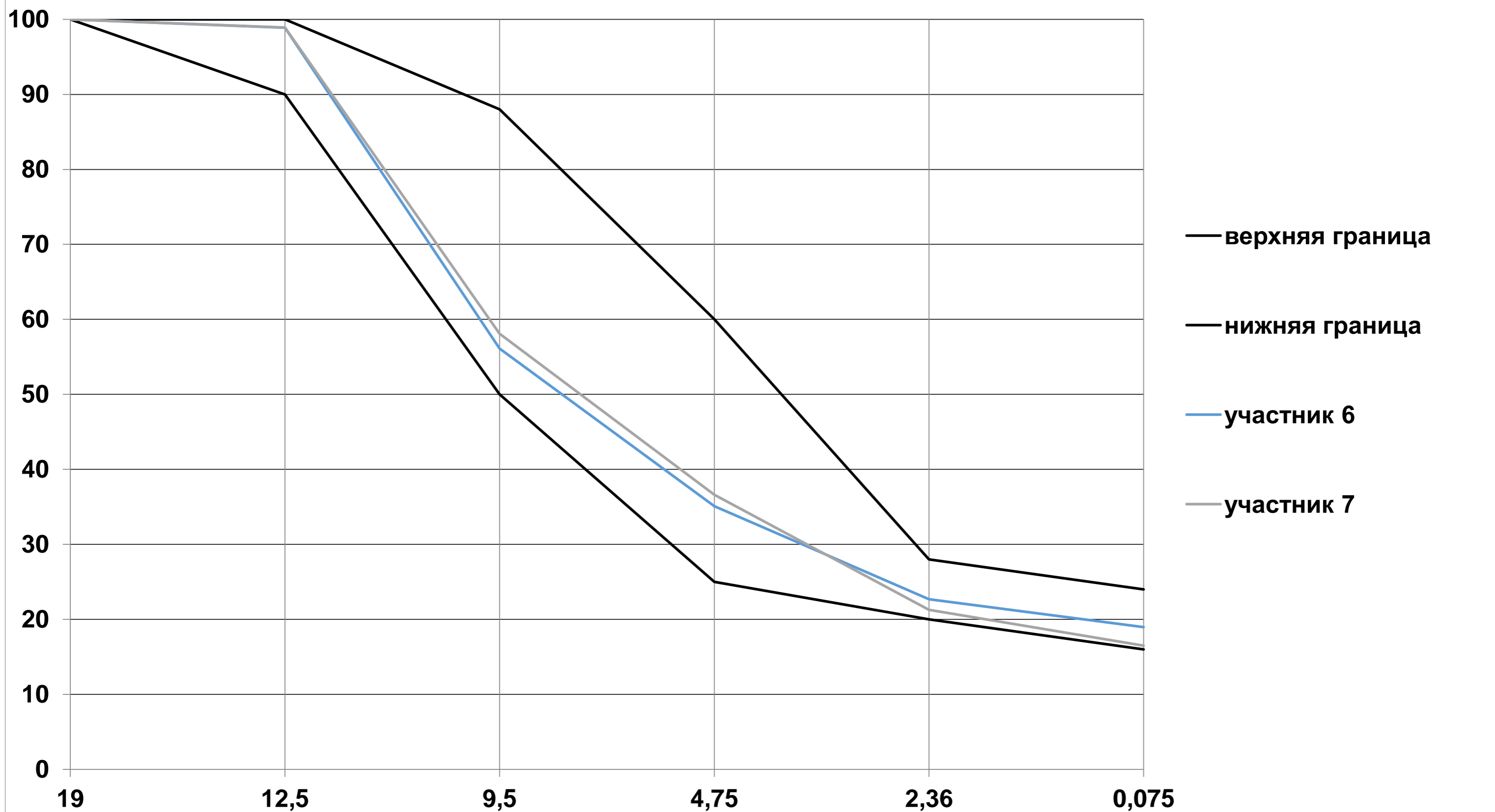
ГОСТ 58401.2. Кривые минеральной части
