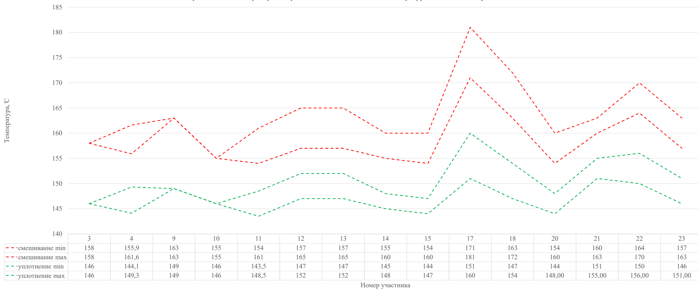
Результаты межлабораторных сравнительных испытаний. Температура смешивания и уплотнения.
